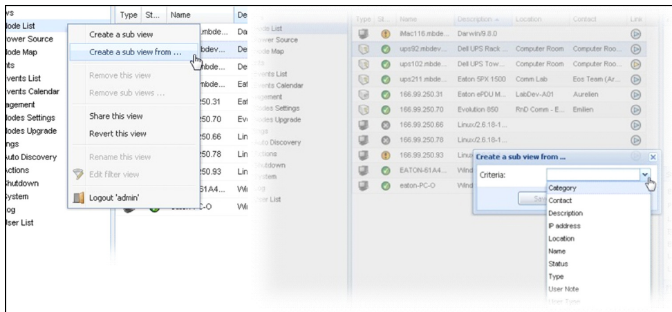
圖 34。子檢視選擇
