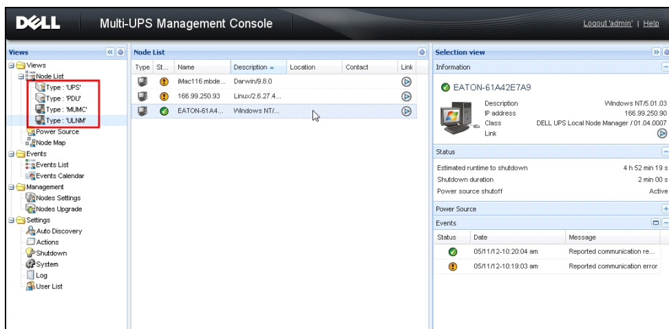
圖 35。示範子檢視
